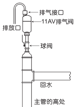
图1 将11AV型自动排气阀安装在系统主管的高处。
